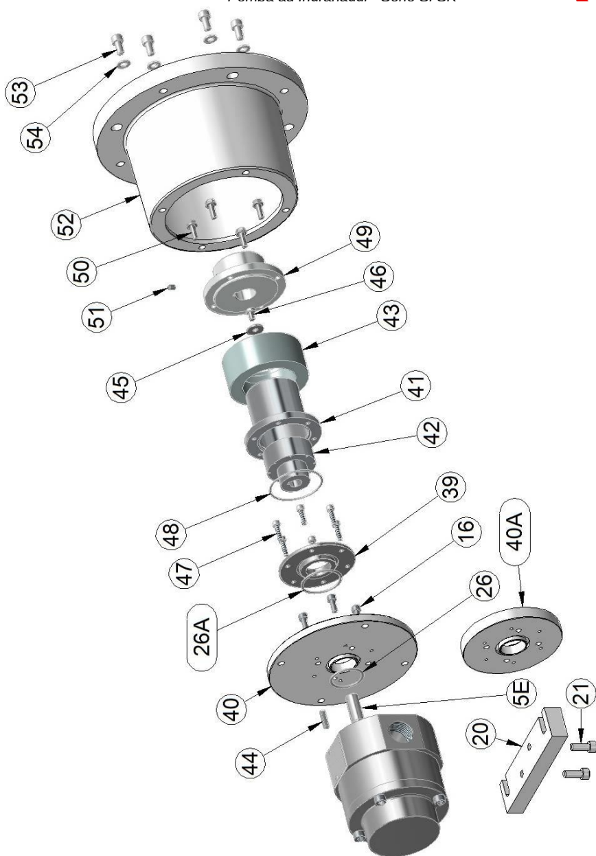
Figura 4 – Giunto magnetico Figure 4 – Magnetic coupling
